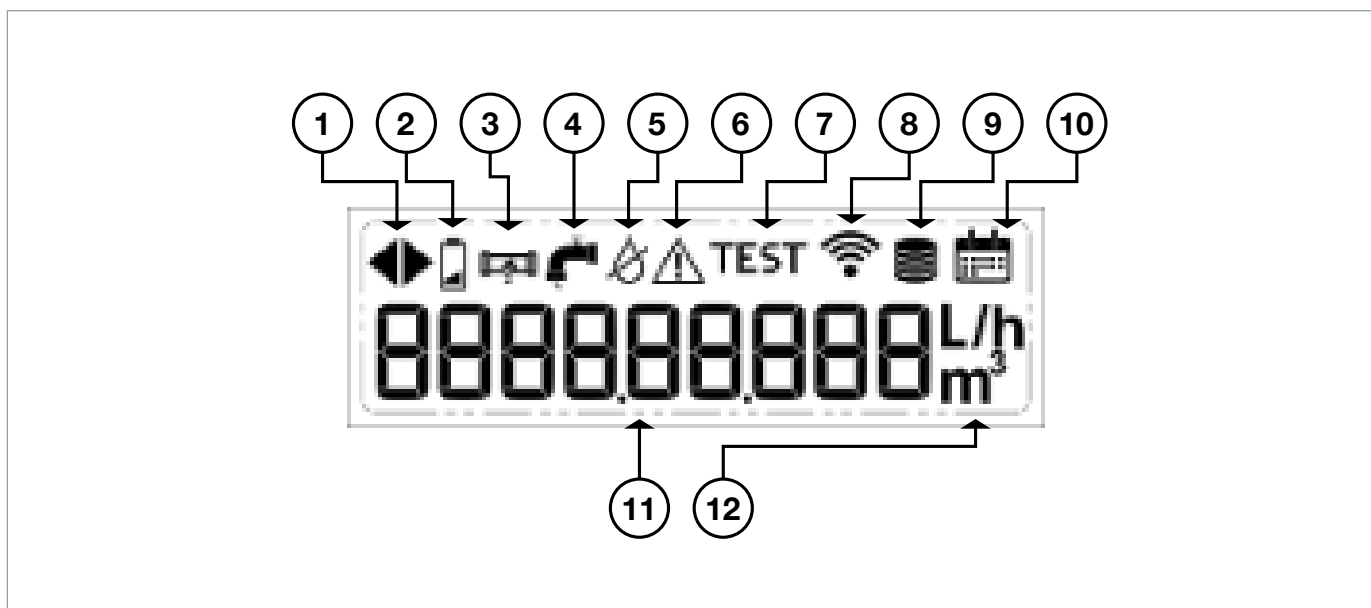
Obr. 5.4. LCD displej SSM-AQUO
