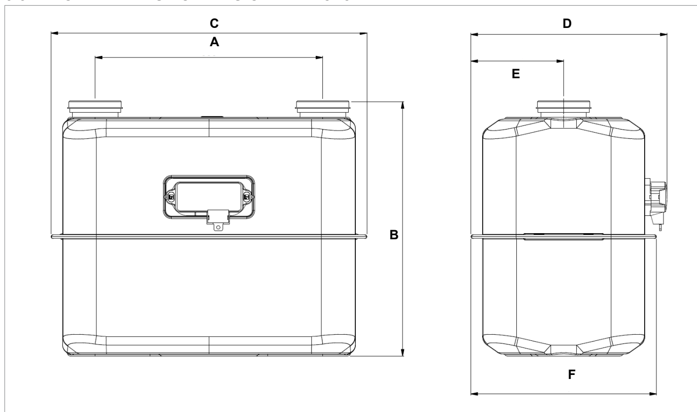
Fig. 6.7. Dimensioni MM int. 335
