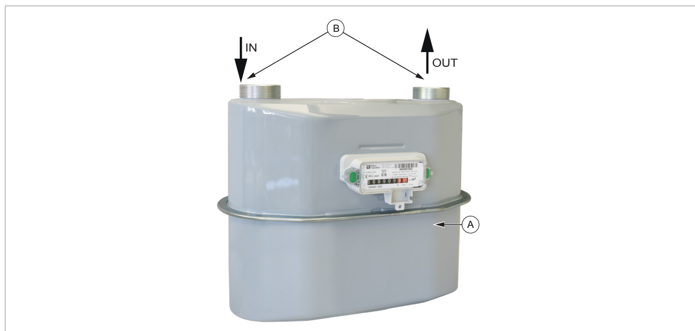
Fig. 7.8. Procedura d'installazione
