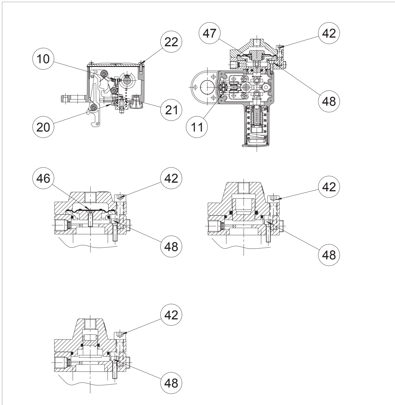
Fig. 9.9. Coppie di serraggio pressostati modelli 102M/102MH ÷ 105M/105MH
