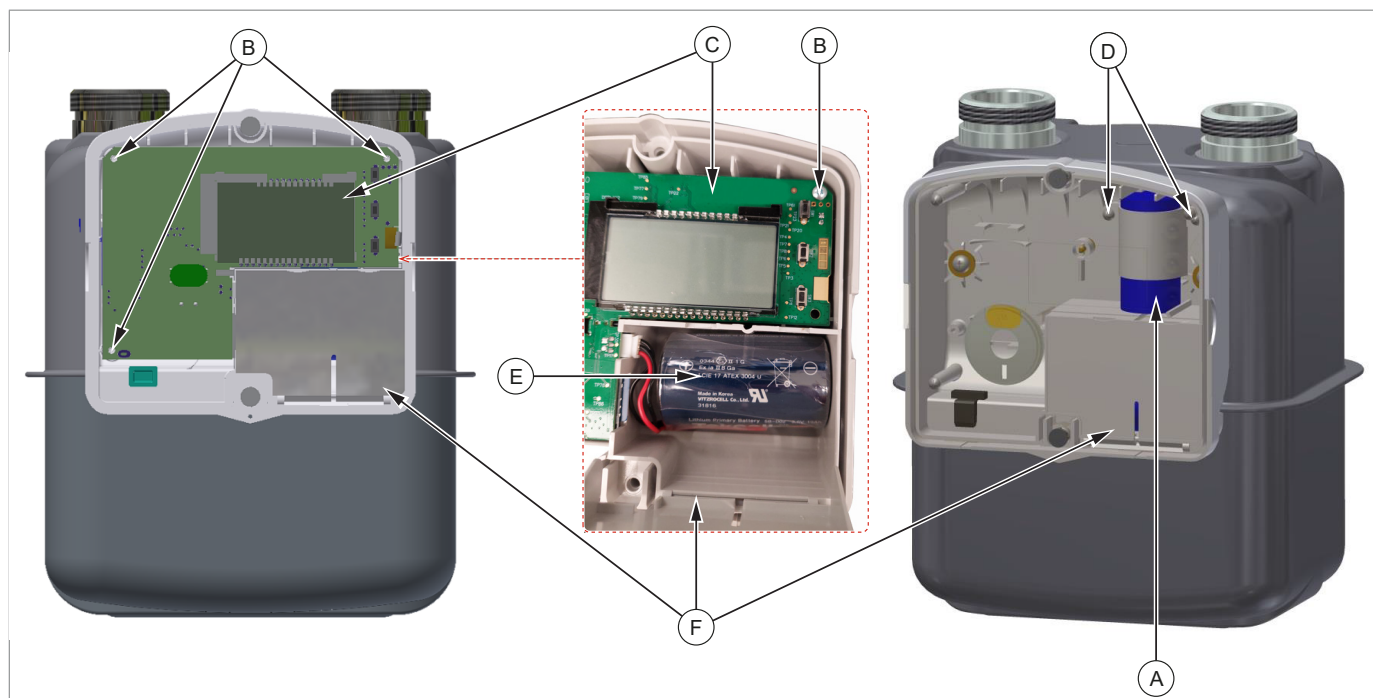
Fig. 10.12. Rimozione batterie
