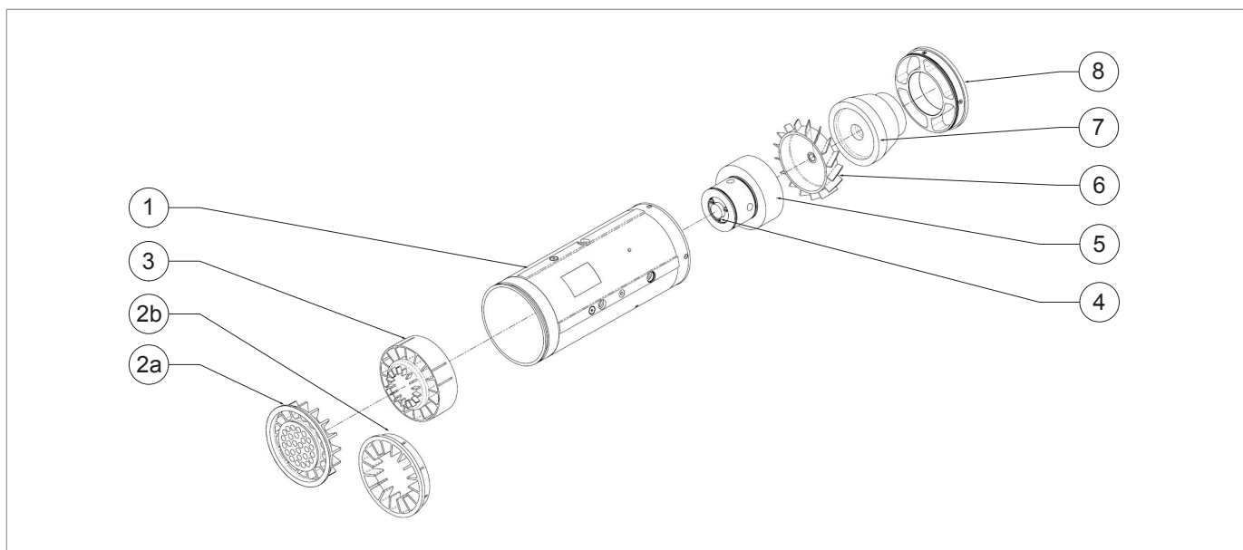
Fig. 4.3. Gruppo cartuccia di misura
