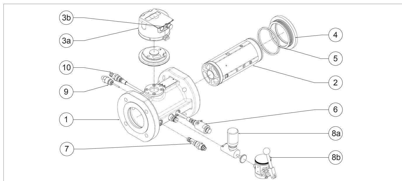
Fig. 4.2. Descrizione generale iM-TM
