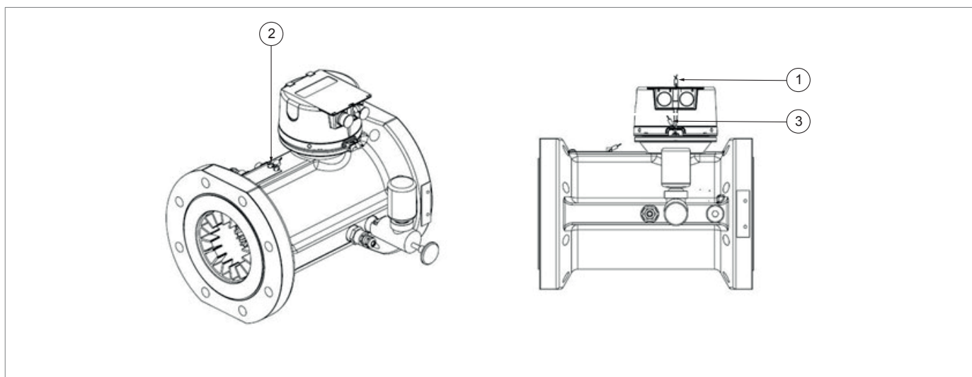
Fig. 4.5. Collocazione sigilli metrologici
